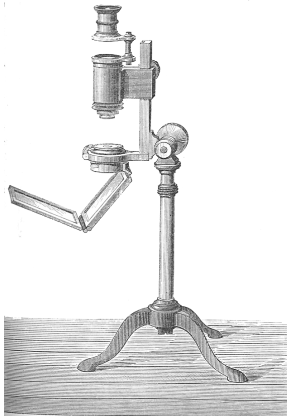
Figure 2. Instrument dérivé du polariscope de Nörremberg, utilisé par Ernest Mallard pour étudier les phénomènes de polarisation en lumière convergente ( in Mallard, 1884) 14 . Un instrument comparable, adapté pour les études en lumière convergente, est exposé au musée de l'École des mines.
