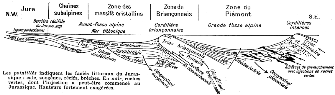
Figure 4. Coupe schématisé indiquant l'aspect que devaient avoir les Alpes françaises vers la fin du Jurassique (inspiré de Wilfrid Kilian et Émile Argand). D'après Gignoux (1950, figure 85).
