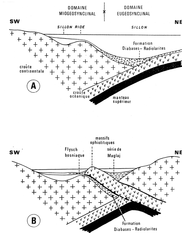
— Le modèle géosynclinal et le paléochariage des massifs ophiolitiques.
