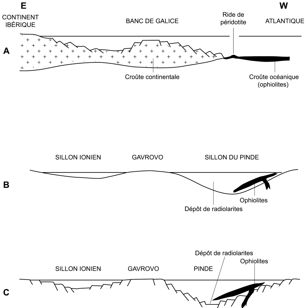
Figure 14. Comparaison de l'ensemble sillon ionien (miogéosynclinal) - haut-fond du Gavrovo (ride miogéantyclinale) - sillon du Pinde à ophiolites (eugéosynclinal) avec la marge actuelle du continent ibérique (bassin - banc de Galice - océan Atlantique).
