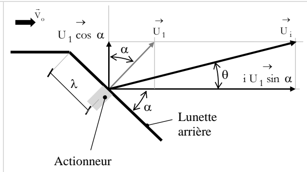
FIG. 14 - Vitesse et orientation du jet pour les échelles 1/N et i/N lorsque la distance \lambda de l'actionneur reste constante, i > 1 .
