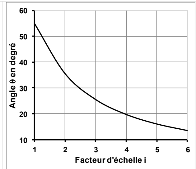
FIG. 16 - Evolutions de l'angle \theta en fonction du facteur d'échelle i , de 1 à N ( N=6 ), lorsque la distance \lambda de l'actionneur par rapport au haut de la lunette arrière reste constante, relation (8).
