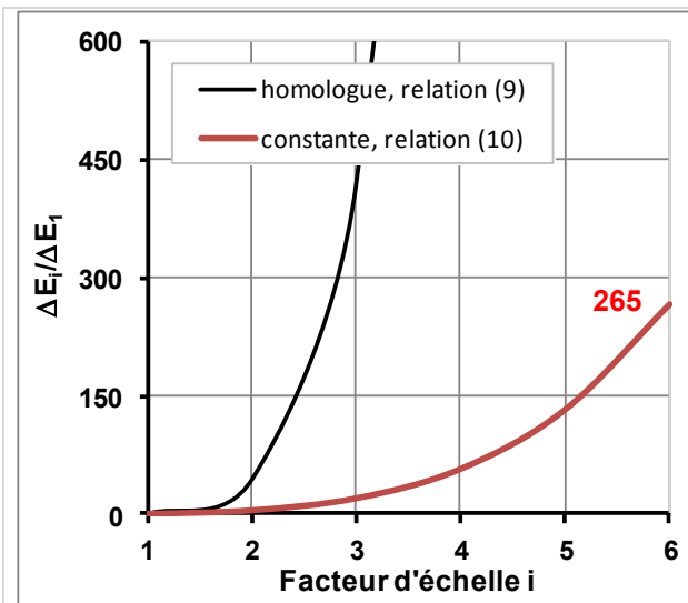
FIG. 17 – Puissances nécessaires au contrôle rapportées à la puissance nécessaire pour l'échelle 1/N ( i=1 et N=6 ) en fonction du facteur d'échelle i (de 1 à N) pour une ligne d'actionneurs positionnée à N\lambda (relation (10)) et \lambda (relation (11)) du haut de la lunette arrière.
