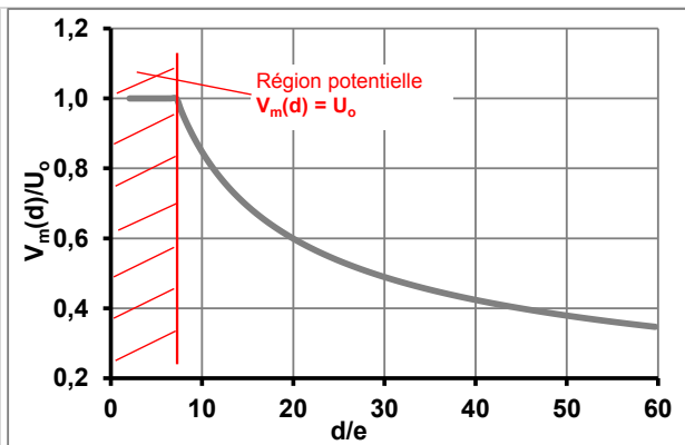
FIG. 12 - Évolution de la vitesse maximale réduite V_m(d)/U_0 relevée dans le plan médian perpendiculaire à la section de sortie de l'actionneur en fonction de la distance réduite d/e , d'après Abramovich (voir la théorie des jets plans [7]).
