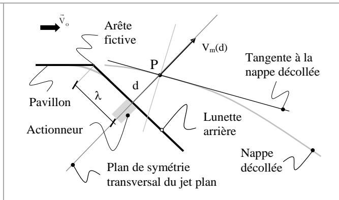
FIG. 2 – Barrette d'actionneurs située à la distance \lambda du haut de la lunette arrière [4-5]. V_m(d) est la vitesse efficace maximale du jet à la distance d de la nappe décollée au plan de la lunette arrière.
