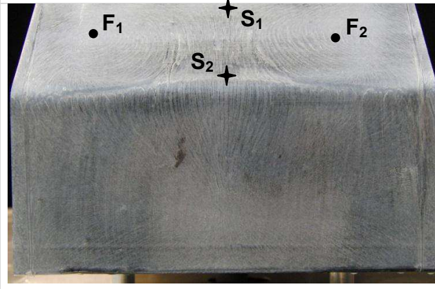
FIG. 6 - Visualisation pariétale sur la lunette arrière et le culot, configuration avec contrôle, [4-5].
