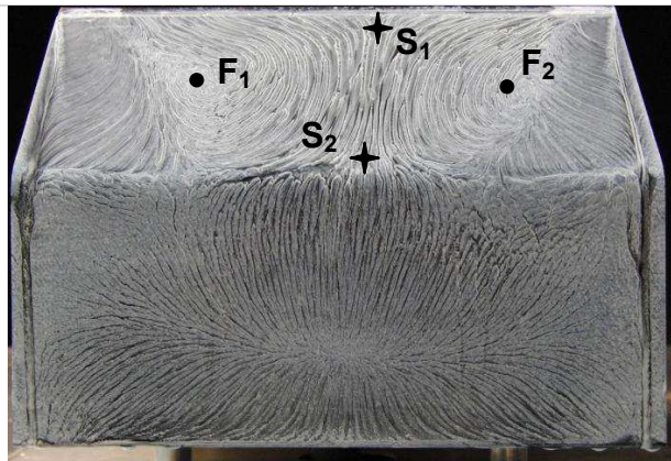
FIG. 5 - Visualisation pariétale sur la lunette arrière et le culot, configuration sans contrôle, [4-5].
