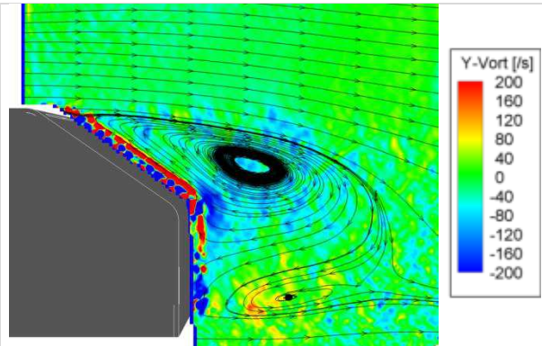
FIG. 4 – Lignes de courant et champ de vorticité suivant y, avec contrôle, [4-5].
