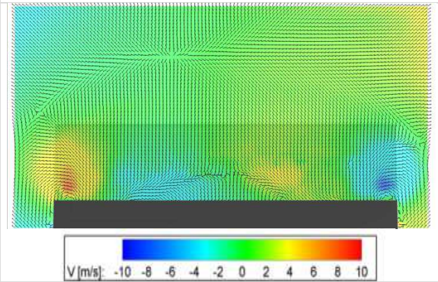
FIG. 8 - Champ de vitesse dans le plan x=2l_A/3 , configuration avec contrôle, [4-5].
