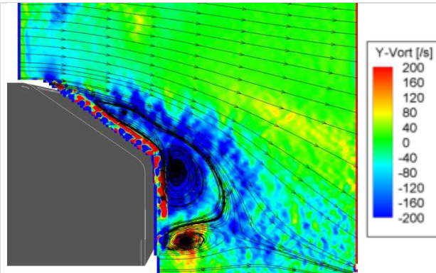
FIG. 3 – Lignes de courant et champ de vorticité suivant y, sans contrôle, [4-5].
