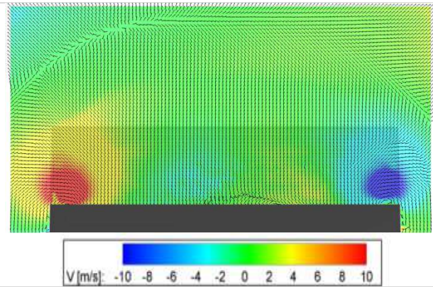
FIG. 7 – Champ de vitesse dans le plan x=2l_A/3 , configuration sans contrôle, [4-5].
