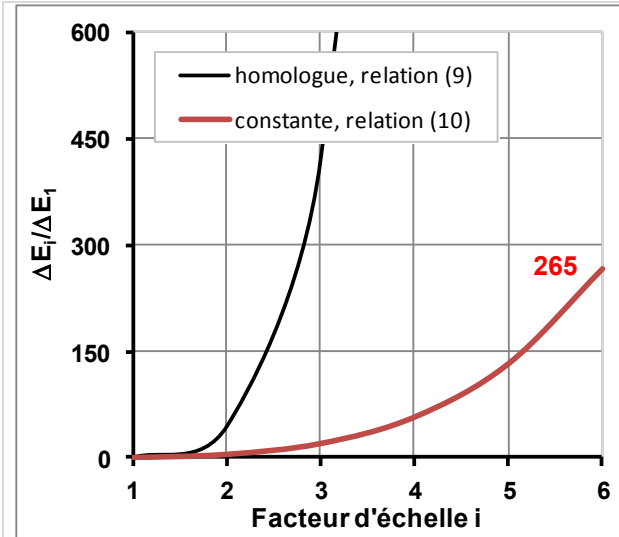
FIG. 17 – Puissances nécessaires au contrôle rapportées à la puissance nécessaire pour l'échelle 1/N ( i=1 et N=6 ) en fonction du facteur d'échelle i (de 1 à N ) pour une ligne d'actionneurs positionnée à N\lambda (relation (9)) et \lambda (relation (10)) du haut de la lunette arrière.
