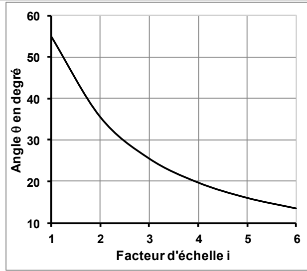
FIG. 16 - Evolutions de l'angle \theta en fonction du facteur d'échelle i , de 1 à N ( N=6 ), lorsque la distance \lambda de l'actionneur par rapport au haut de la lunette arrière reste constante, relation (8).
