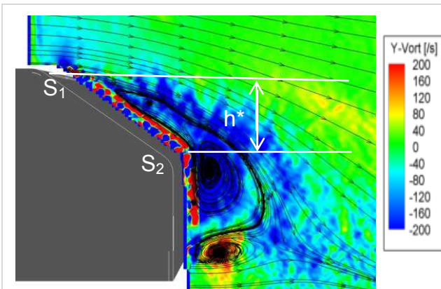
FIG. 9 – Lignes de courant et champ de vorticit  sans contr le [4,5]. Les traits blancs représentent les traces des deux plans horizontaux qui passent par les points selle S_1 et S_2 rep r s sur les figures 5 et 10.
