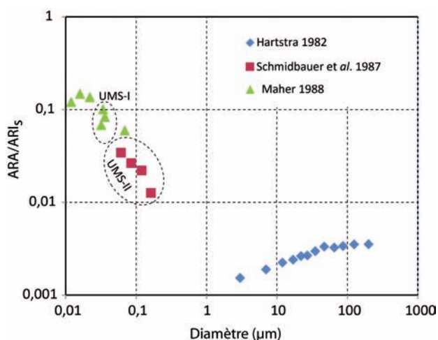
Fig. 6—Le rapport de ARA/ARI s en fonction du diamètre des grains de magnétite (μm).
