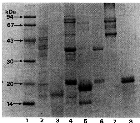
Fig 1. SDS-PAGE electrophoresis of MW standards (lane 1), raw lupin flour (lane 2), the lupin concentrate (lane 3), raw soyabean flour (lane 4), the soyabean concentrate (lane 5), and purified glycinin (lane 6), \beta -conglycinin (lane 7) and \alpha -conglycinin (lane 8).
