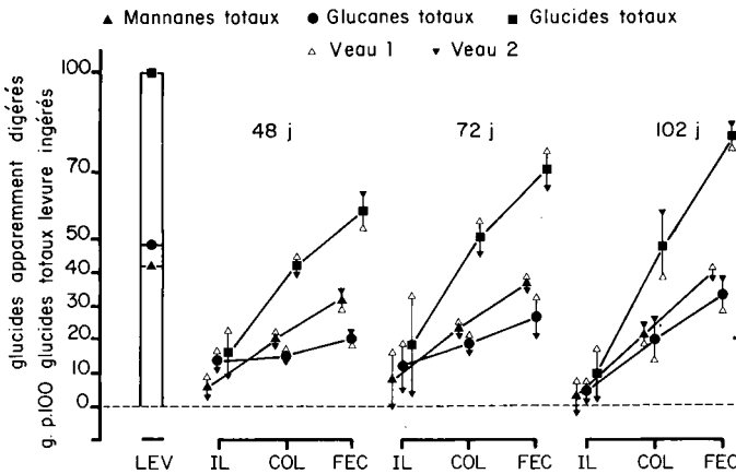
FIG. 3. — Quantités de glucides apparemment digérées le long du tube digestif (g p. 100 g de la somme des glucides de levure ingérés). LEV = levure ; IL = iléon ; COL = côlon ; FEC = fèces.
