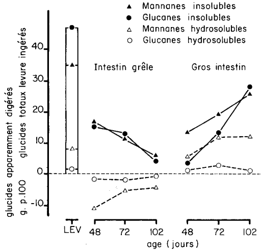
FIG. 5. — Evolution avec l'âge de la digestion des glucides (g p. 100 de la somme des glucides de levure ingérés, Veau n° 2). LEV = levure.
