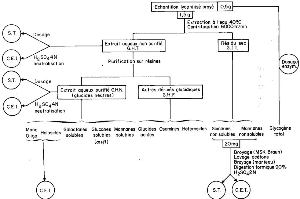
FIG. 1. — Fractionnement glucidique. C.E.I. = analyse par chromatographie échangeuse d'ions ; S.T. = dosage des sucres totaux ; G.H.T. = glucides hydrosolubles totaux ; G.H.F. = glucides hydrosolubles fixés par purification ; G.H.N. = glucides hydrosolubles neutres ; G.I.T. = glucides insolubles totaux.
