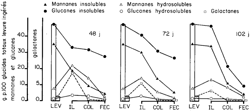
FIG. 4. — Evolution de la digestion des glucides dans le tube digestif (g p. 100 g de la somme des glucides levure ingérés, Veau n° 2).
