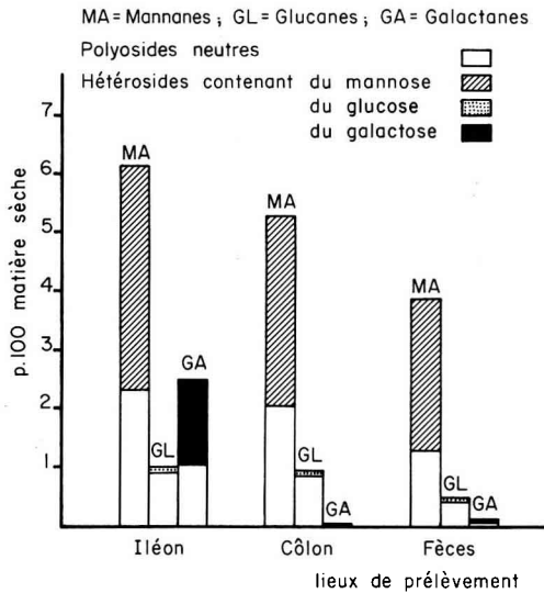
FIG. 2. — Composition en polyosides neutres et en hétérosides des extraits aqueux (Veau n° 1, 48 jours).
