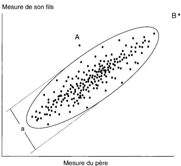
Figure 1. Principe de l'estimation d'une covariance entre apparentés. Chaque point représente un couple de mesures d'un père et de son fils. La covariance mesure l'étirement du nuage de points, elle est inversement liée à l'épaisseur "a".
