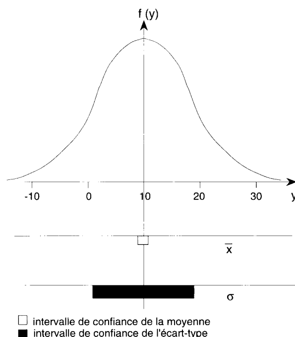
Figure 2. Longueur des intervalles de confiance pour l'estimation d'une moyenne et d'un écart-type. L'estimation porte sur un échantillon de 40 données y , tirées de la population de moyenne 10 et d'écart-type 10 représentée au-dessus.
