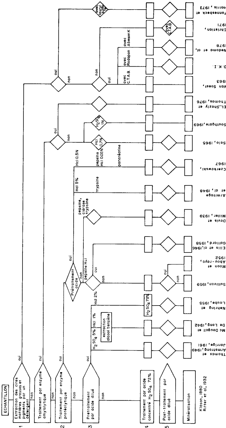
FIG. 3 Schéma de base des méthodes basées sur un traitement à l'acide sulfurique concentré (lignes de Klaton). Methods based on treatment with concentrated sulfuric acid (Klaton lignin).
