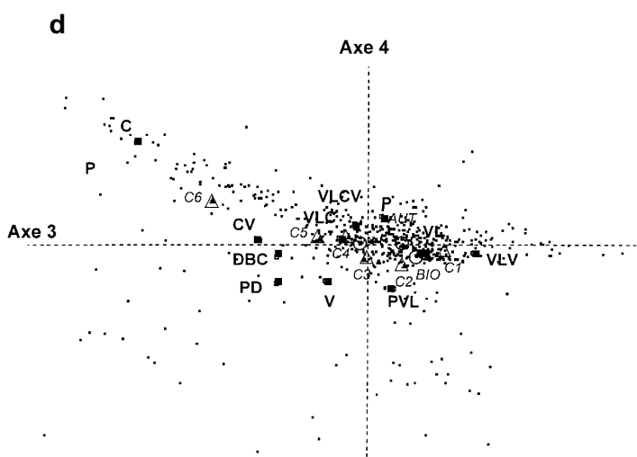
Figure 3. Analyse en composantes principales sur le tableau des données relatives aux bilans d'azote des 555 exploitations agricoles enquêtées : plan principal représentant les variables (a) et les individus (b) ; plan des axes 3 et 4 représentant les variables (c) et les individus (d).
