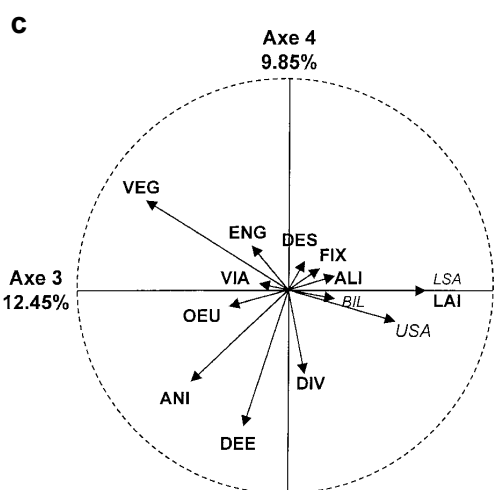
Figure 3. Analyse en composantes principales sur le tableau des données relatives aux bilans d'azote des 555 exploitations agricoles enquêtées : plan principal représentant les variables (a) et les individus (b) ; plan des axes 3 et 4 représentant les variables (c) et les individus (d).
