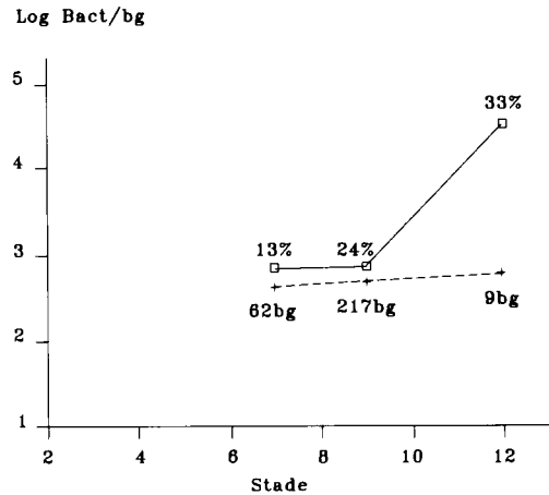
Fig 6. Comparaison des teneurs en bactéries de bourgeons gelés ( \square-\square ) ou non gelés ( +--+ ) au seuil de -3,5^{\circ}\text{C} . Les chiffres indiquent le pourcentage de bourgeons gelés et le nombre total analysé à un stade donné.
