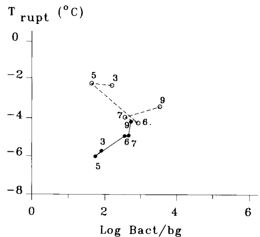
Fig 4. Évolution de la moyenne des températures de rupture de surfusion en fonction de la teneur en bactéries par bourgeon et du stade phénologique selon que les bourgeons de Chardonnay sont secs (●) ou mouillés (○). Les chiffres indiqués correspondent aux numéros des stades phénologiques.
