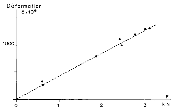
Figure 7 Déformation de la fibre du tronc à la hauteur H 1 = 1 m sous l'action d'un effort horizontal.
