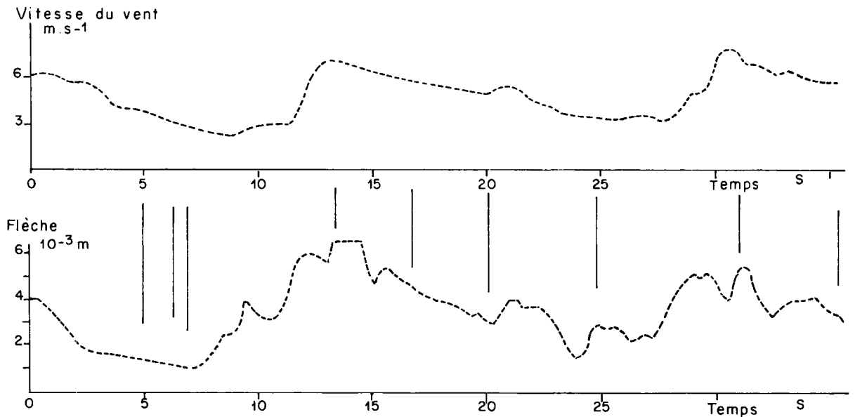
Figure 8 Enregistrements simultanés de la vitesse du vent et de la flèche d'un arbre à la hauteur H_1 = 0,73 m.
