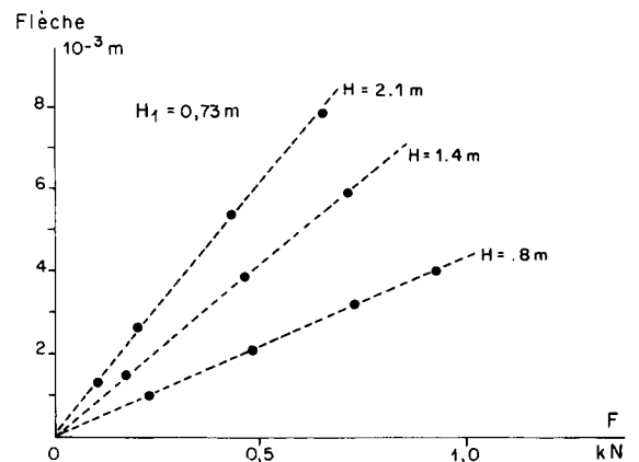
Figure 6 Méthode du chariot : fléchissement d'un arbre en fonction de l'effort horizontal. Waggon method : tree bending versus horizontal force.
