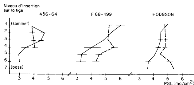
Figure 2 Effet du déficit hydrique sur le poids spécifique du limbe (PSL, mg/cm 2 ), en fonction du niveau d'insertion sur la tige. Drought stress effect on specific leaf weight (PSL, mg/cm 2 ) according to the leaf position on the stem.
