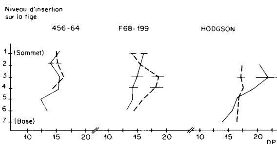
Figure 5 Effet du déficit hydrique sur la densité du parenchyme palissadique (DP, en nombre de cellules par unité de longueur de coupe) en fonction du niveau d'insertion sur la tige. Drought stress effect on palisade parenchyma (DP, number of cells/length unit) according to leaf position on the stem.
