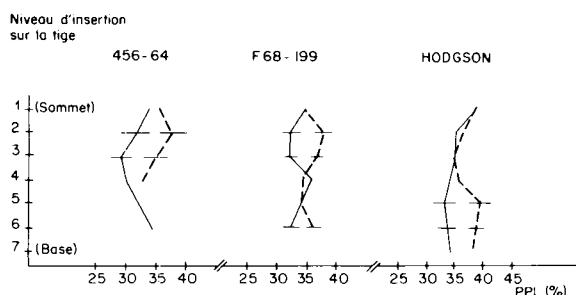
Figure 4 Effet du déficit hydrique sur la proportion de parenchyme lacuneux (PPL, en p. 100) en fonction du niveau d'insertion sur la tige. Drought stress effect on spongy parenchyma ratio (PPL, %) according to leaf position on the stem.
