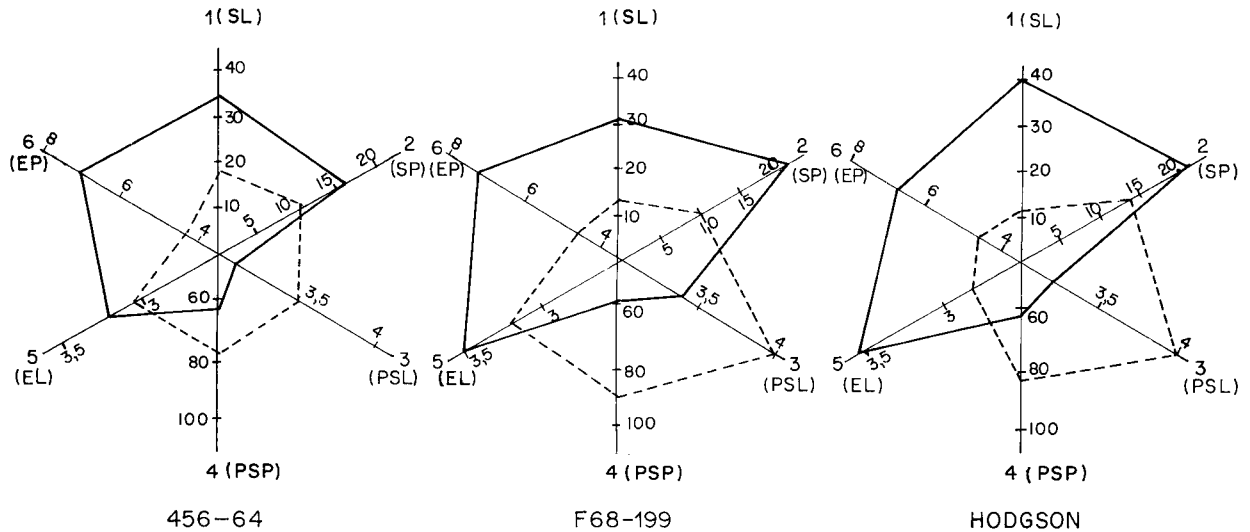
Figure 1 Effet du déficit hydrique sur quelques caractères des feuilles en cours de croissance : surface du limbe (SL, cm 2 ) et de la section du pétiole (SP, mm 2 ), poids spécifique du limbe (PSL, mg/cm 2 ) et du pétiole (PSP, mg/cm 3 ), teneur en eau du limbe (EL, mg eau/mg matière sèche) et du pétiole (EP, mg eau/mg matière sèche).
