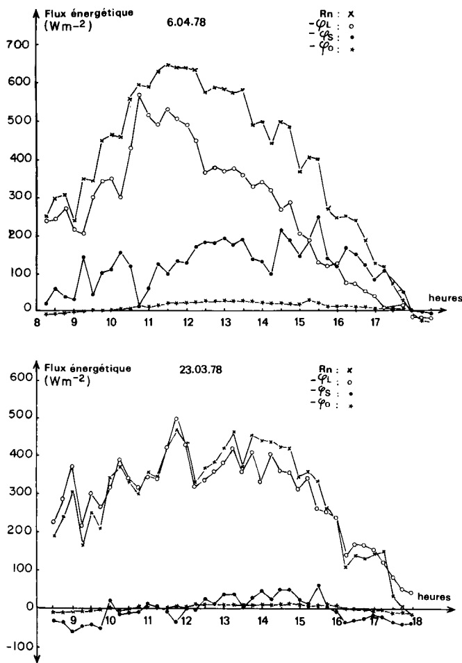
Figure 3 Exemples d'évolution journalière des différents termes du bilan d'énergie dans le cas du gazon. Typical daily changes in the different components of the energy balance for lawn.
