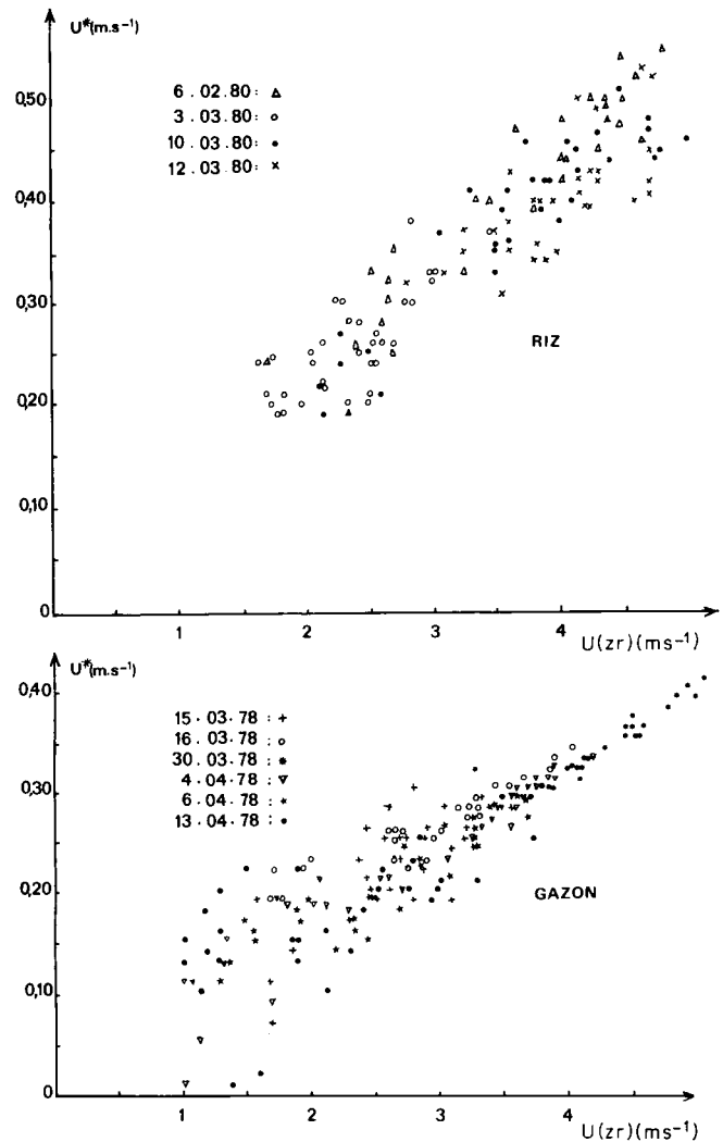
Figure 2 Evolution de la vitesse de frottement u_x en fonction de la vitesse du vent au niveau de référence ( z_r ) : a) cas du riz ( z_r = 3 m). b) cas du gazon ( z_r = 2,5 m). Friction velocity u_x as a function of wind speed at a reference level ( z_r ) : a) for the rice crop ( z_r = 3 m). b) for the lawn ( z_r = 2,5 m).
