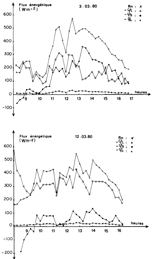
Figure 4 Exemples d'évolution journalière des différents termes du bilan d'énergie dans le cas du riz (avant irrigation le 3 mars et après irrigation le 12 mars). Typical daily changes in the different components of the energy balance for the rice crop (3 march : before irrigation ; 12 march : after irrigation).
