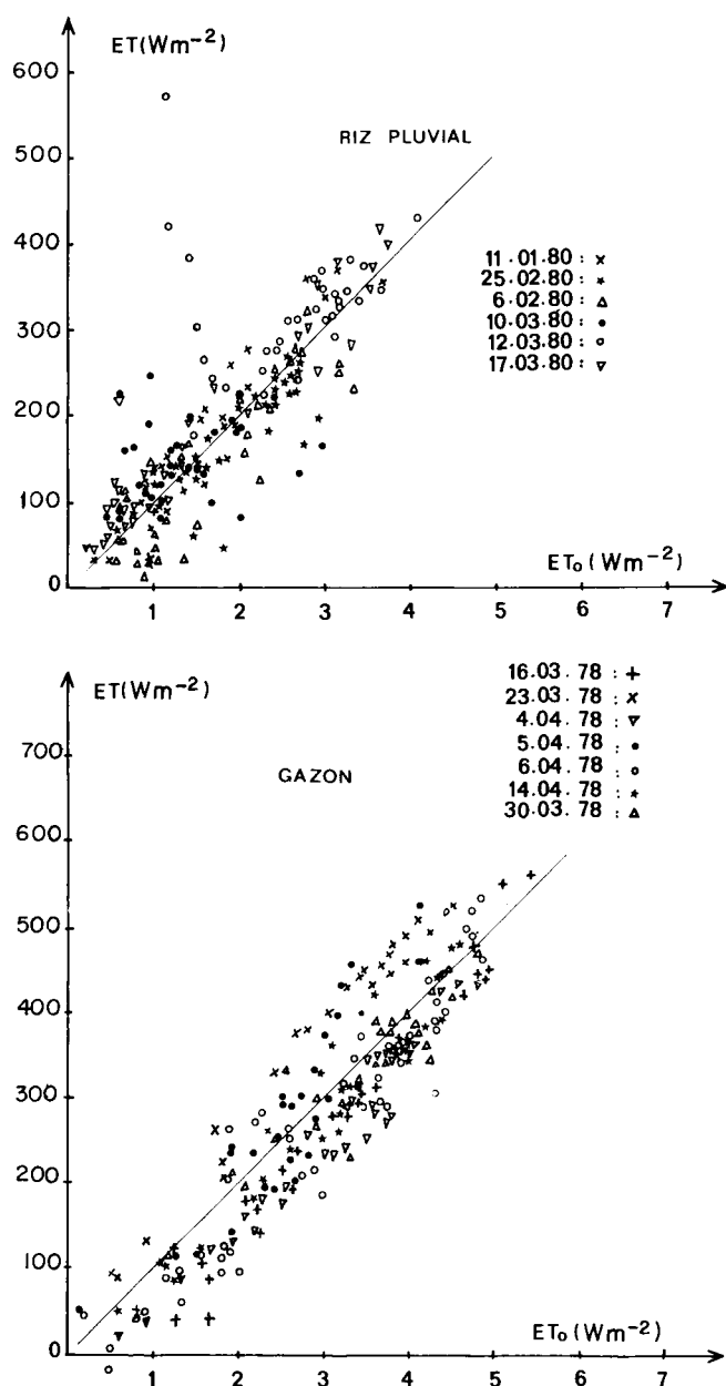
Figure 5 Evapotranspiration réelle (ET) en fonction de l'évapotranspiration standard ( ET_0 ) :
