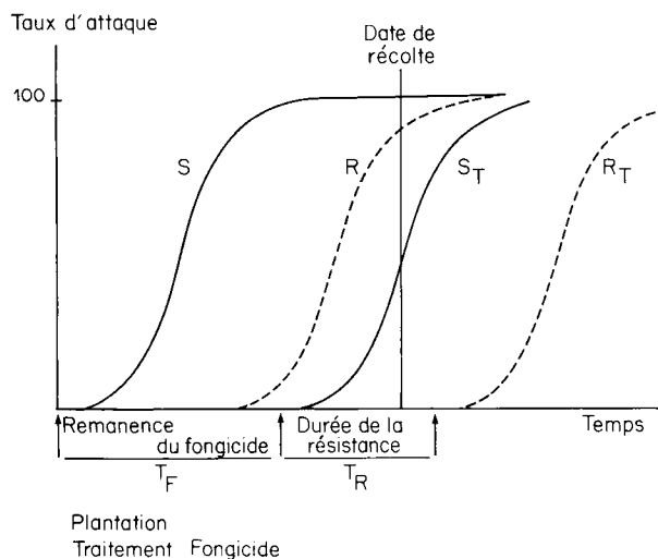
Figure 1 Courbes d'évolution théoriques d'une épidémie chez une variété sensible (—) et une variété résistante (- - -) traitées ( S_T et R_T ) ou non traitées ( S et R ) à l'aide d'un fongicide rémanent.
