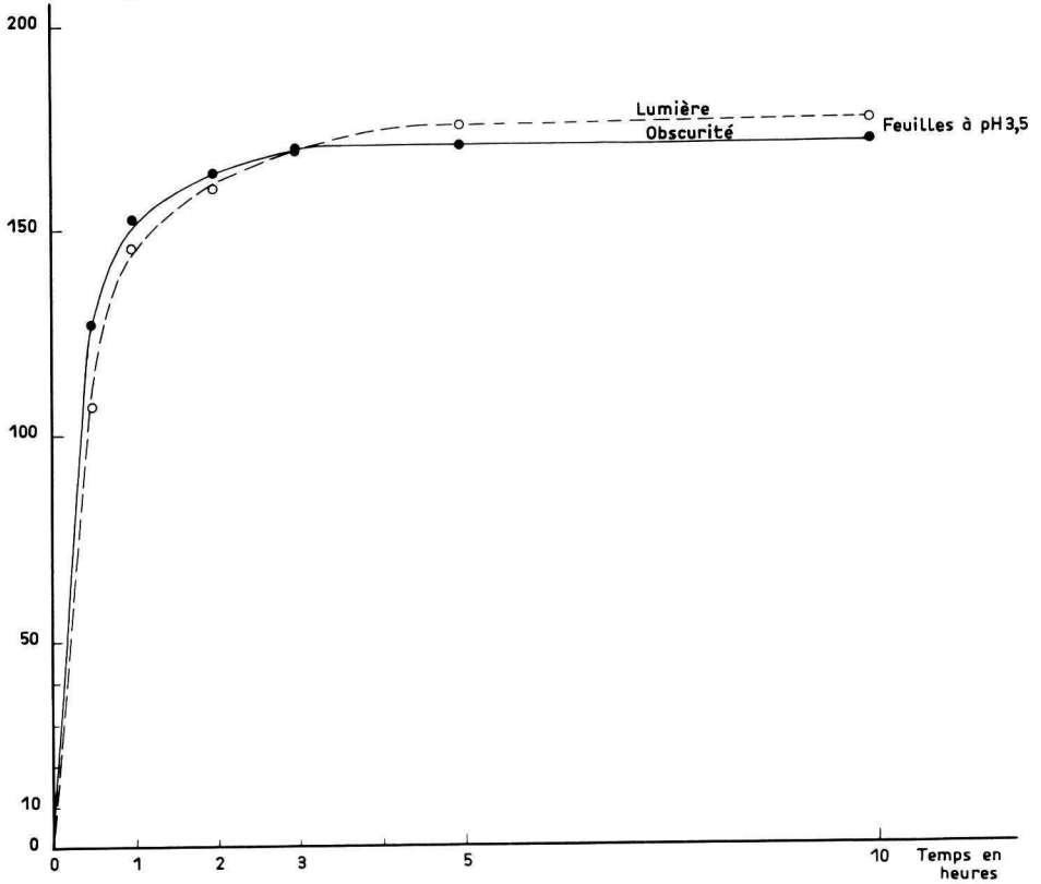
FIG. 4. — Réduction des nitrites par voie non enzymatique : influence de la lumière et de l'obscurité. Pinus nigra laricio (corsicana), 2 ans, aiguilles pH 3,5
