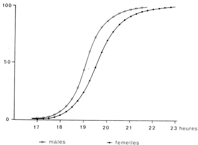
FIG. 4. — Sorties horaires des adultes de Th. pityocampa. Courbes de fréquences cumulées par sexe (de quart d'heure en quart d'heure, sur 4 000 adultes). Population du Mont Ventoux : altitude de 500 m.
