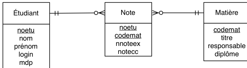
FIGURE 2: Exemple de "Crow's Foot Diagram" pour le modèle relationnel
