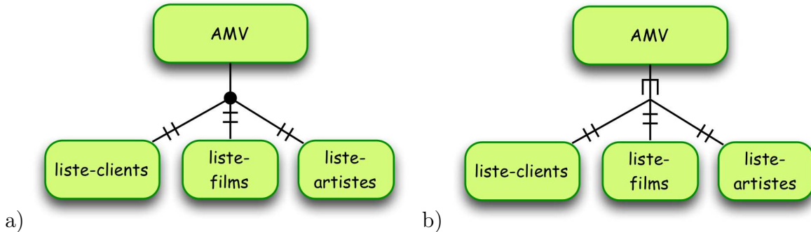
FIGURE 10: Composition d'éléments (a) en séquence et (b) en alternative
