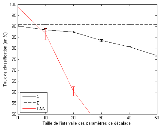
FIGURE 3 – Taux de classification \bar{\eta}_{consist} sur les vecteurs de caractéristiques extraits des signaux traduits aléatoirement par les fonctions de groupement \Sigma(\cdot) et \Sigma'(\cdot) , et pour le CNN.
