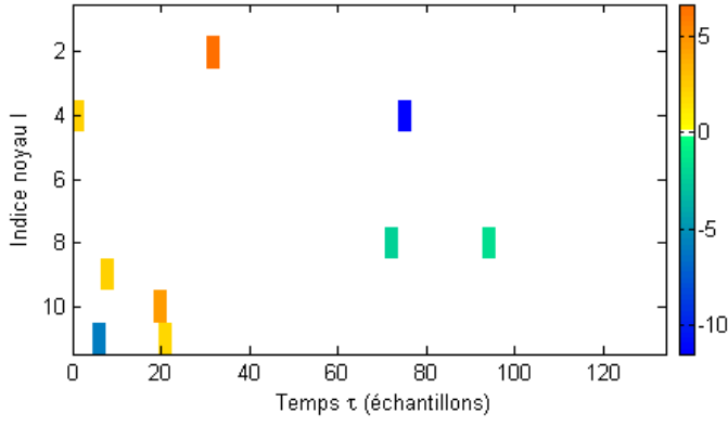
FIGURE 1 – Spikegramme de la lettre e où l'amplitude (couleur) des coefficients x_{l,\tau} est représentée en fonction du temps \tau (abscisse) et de l'indice du noyau l (ordonnée).
