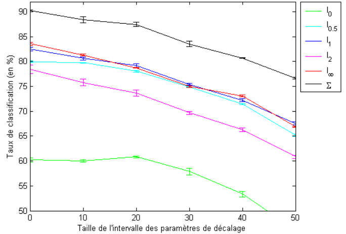
FIGURE 2 – Taux de classification \bar{\eta}_{consist} sur les vecteurs de caractéristiques extraits des signaux traduits aléatoirement pour les fonctions de groupement fenêtrées.
