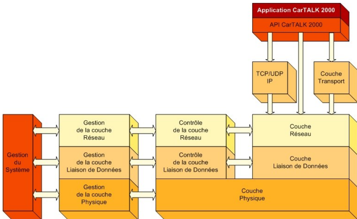
Figure 4. Architecture du protocole CarTALK (adapté depuis [9])
