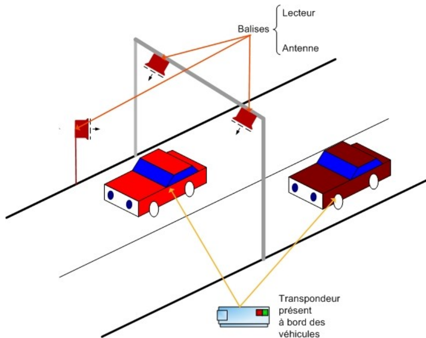
Figure 1. Principe de fonctionnement du protocole DSRC [10].
