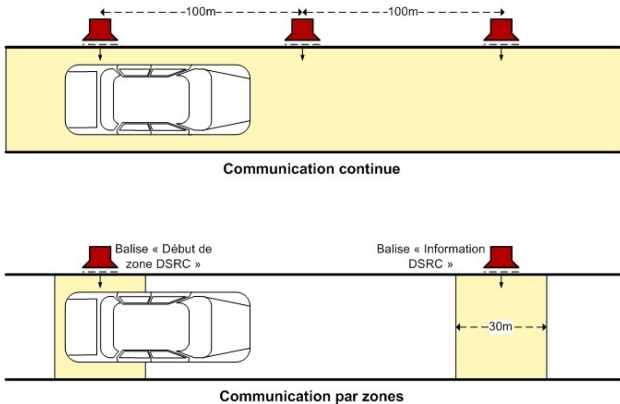
Figure 3. Communication continue et communication par zones [10].
