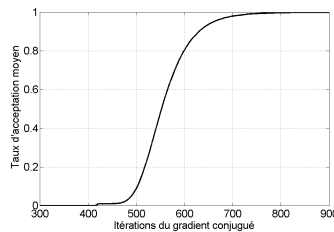
FIGURE 1 – (Gauche) comparaison des méthodes en terme de moyenne et d'écart-type des paramètres estimés ; (Droite) taux d'acceptation moyen en fonction du nombre d'itérations du gradient conjugué.
