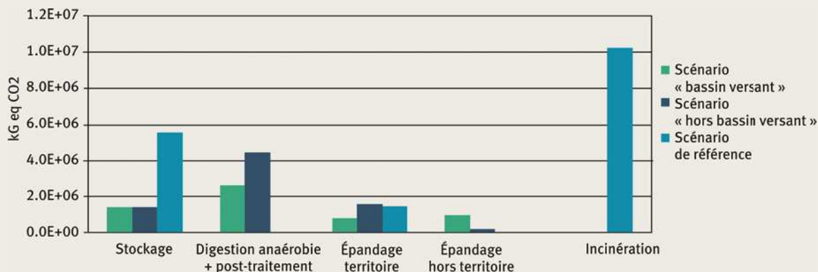
7 Comparaison des trois scénarios pour l'impact changement climatique.
