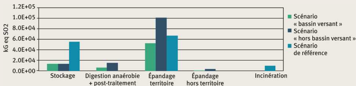
6 Comparaison des trois scénarios pour l'impact eutrophisation.
