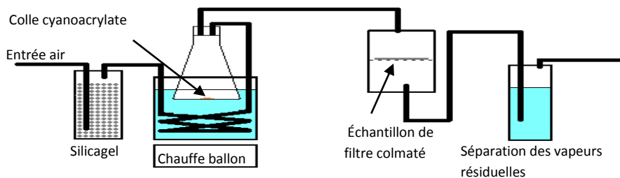
Figure 4 : dispositif de fixation des filtres colmatés (Schmidt, 1990)
