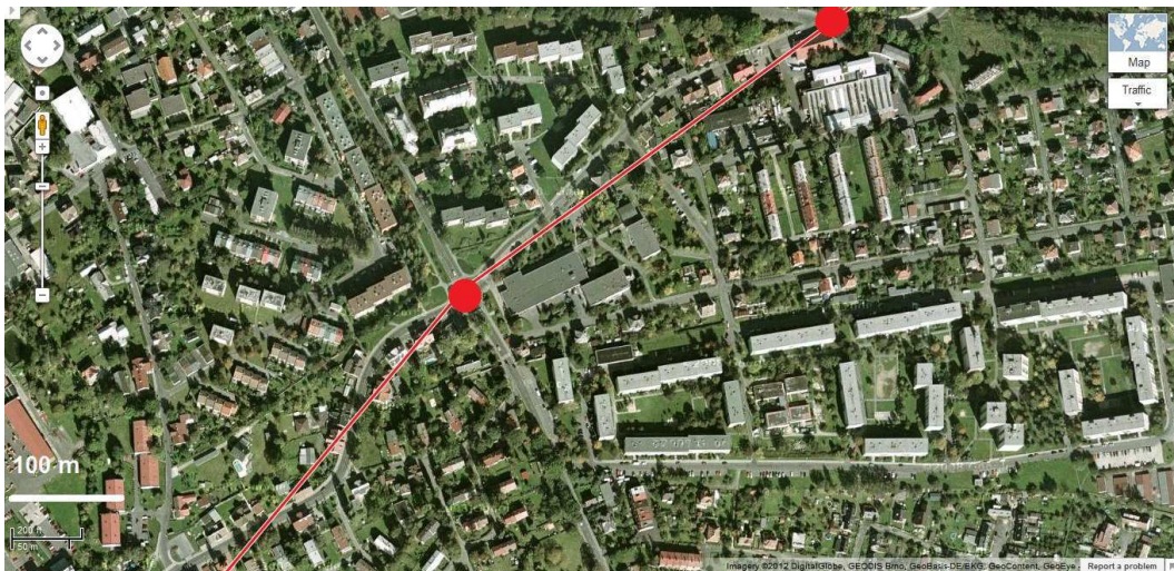
Figure 26 : Le tramway à Liberec dessert environ la moitié des ensembles de logement collectif à l'échelle de la ville, ici une esquisse indicative (source : auteur sur le support de www.dpml.cz ).
