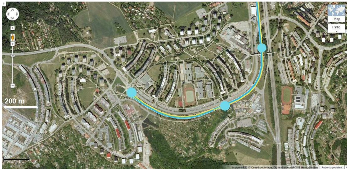
Figure 31 : Le tramway à Brno dessert environ la moitié des ensembles de logement collectif à l'échelle de la ville, ici une esquisse indicative (source : auteur sur le support de www.idsjmk.cz ).
