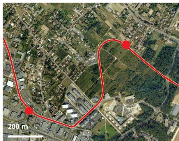
Figure 22 : Le choix du tracé du tramway autour de la Lorette suscite des questions (source : auteur sur le support de GoogleMaps).
