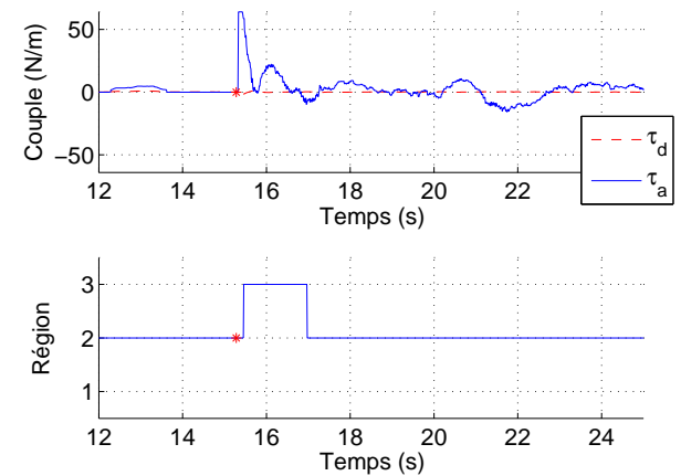
FIGURE 7. Couple conducteur et couple d'assistance (entrée de commande) pendant l'évitement de sortie de voie.
