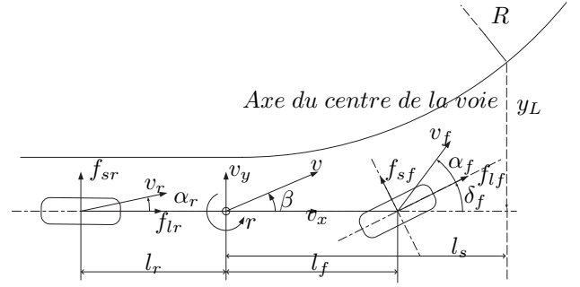
FIGURE 2. Modèle bicyclette du véhicule
