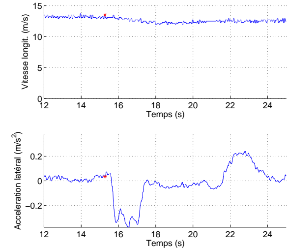
FIGURE 6. Vitesse longitudinale et accélération latérale pendant l'évitement de sortie de voie.
