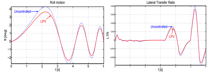
Fig. 12. Roll motion \theta .
