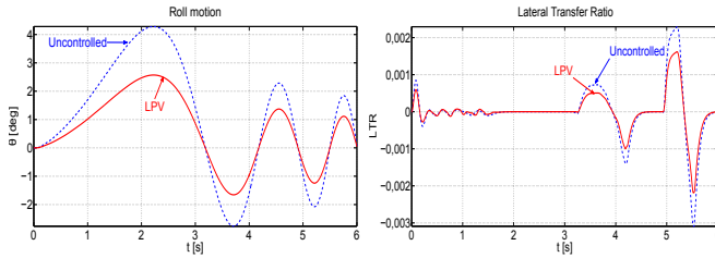
Fig. 20. Roll motion \theta .
