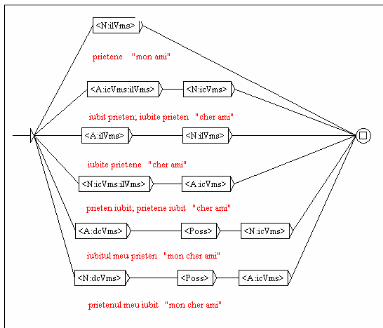
Figure 3. Conditionnement syntaxique
