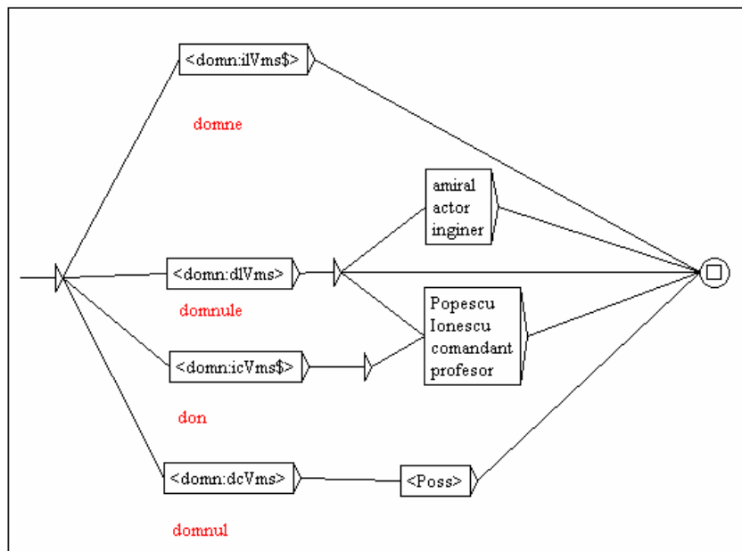
Fig. 2. Conditionnement phonético-syntaxique
