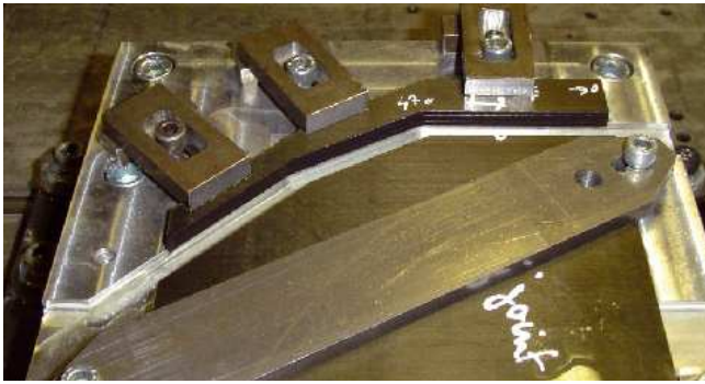
Fig. 3. Dispositif expérimental.
