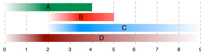
FIGURE 15 – Une représentation des processus A, B, C, D utilisant des dégradés de couleur pour rendre compte des incertitudes.
