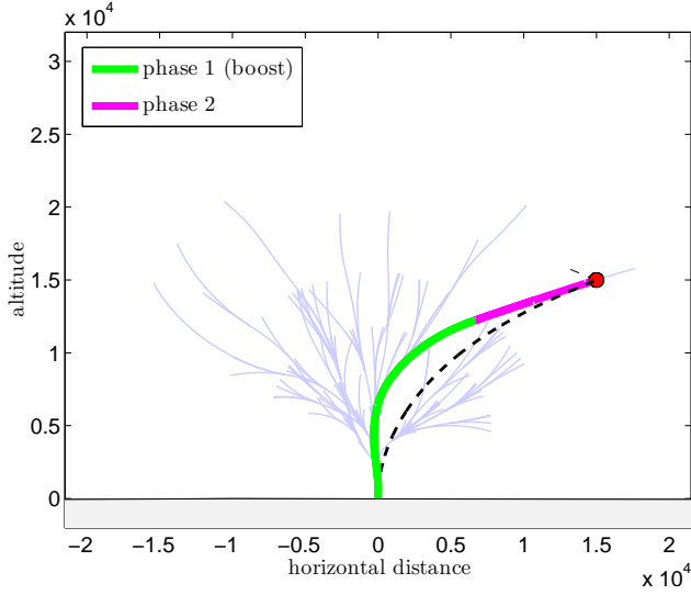
Fig. 6. Scenario 1 - Trajectories
