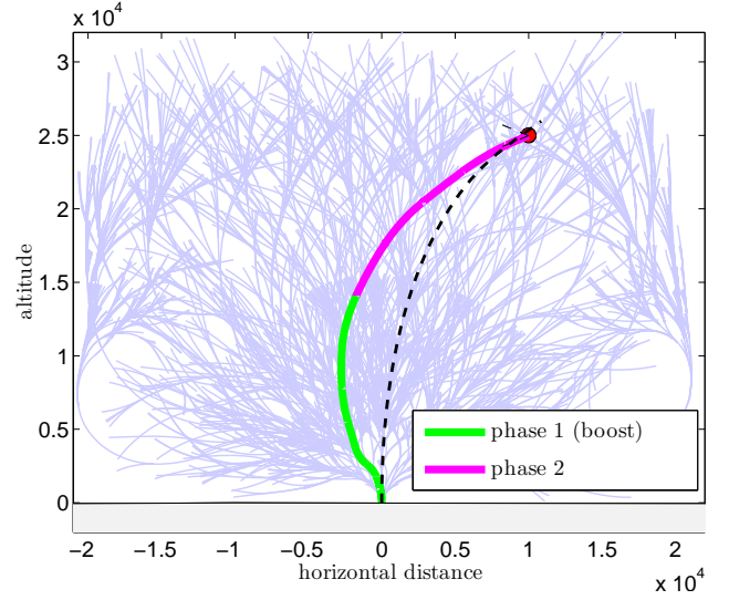
Fig. 8. Scenario 2 - Trajectories
