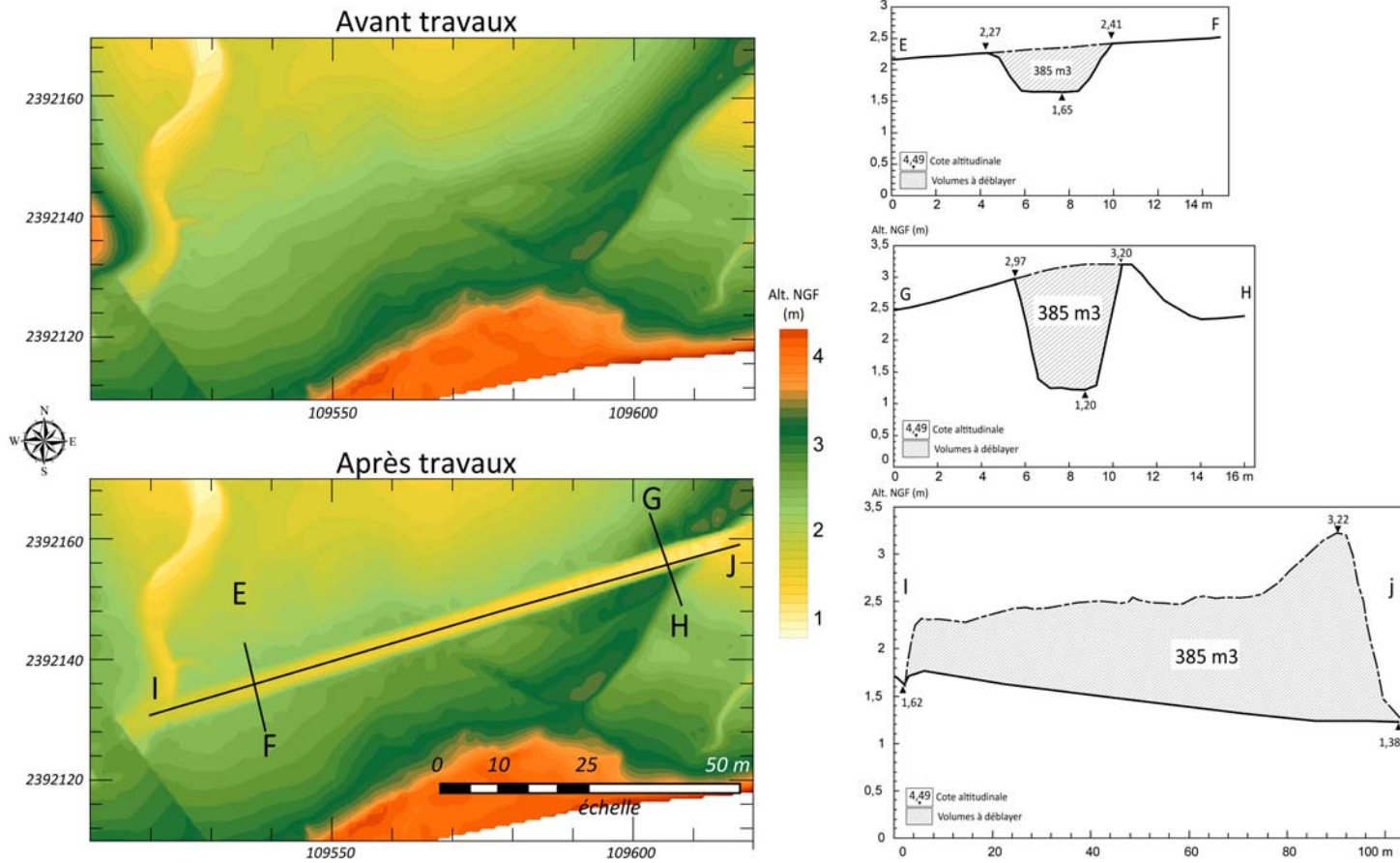
Figure 22 – Profils topographiques et cotes altitudinales avant et après l'ouverture d'un nouveau chenal (étape 3).
