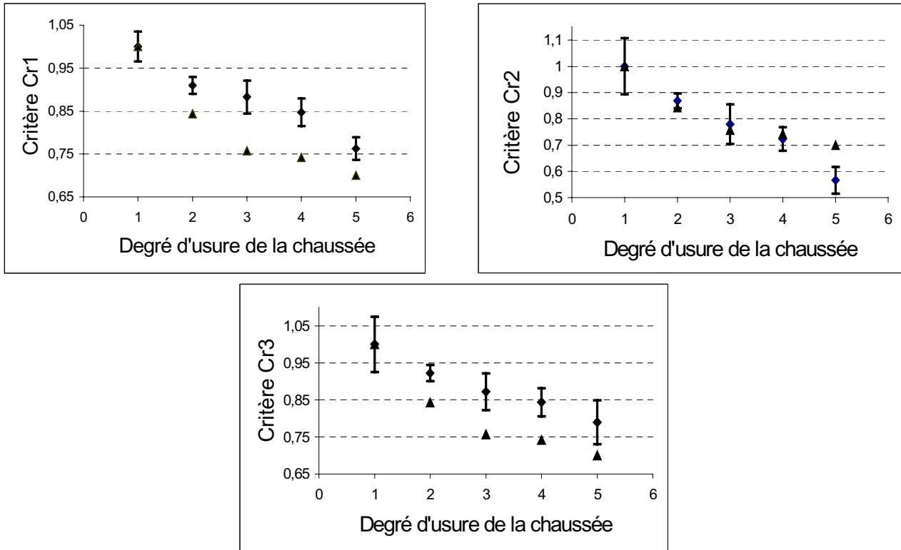
Figure 5. Evolution des critères de rugosité (◆) et du critère SRT (▲) en fonction du degré d'usure
