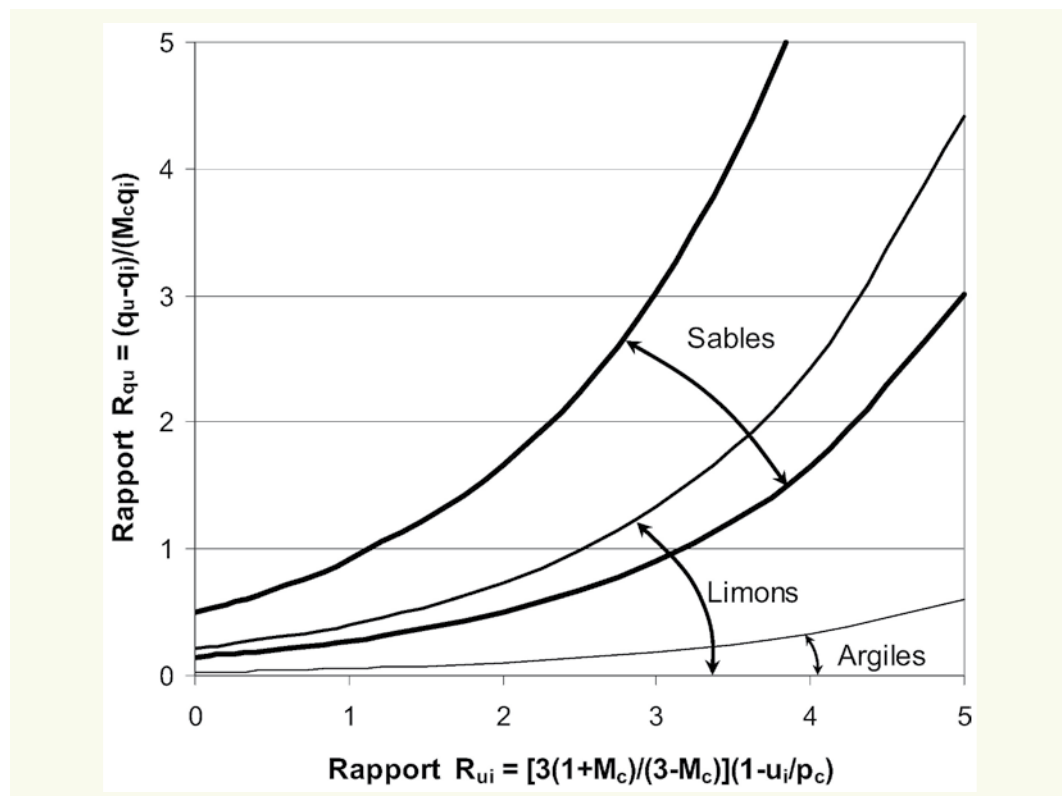
figure 5 Identification des types de sols d'après la valeur des coefficients d'élongement des chemins de contraintes des essais de compression consolidés non drainés à l'appareil triaxial
