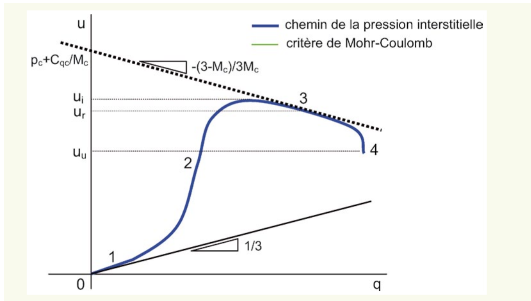
figure 2 Évolution du déviateur q et de la pression interstitielle u dans un essai de compression consolidé non drainé à l'appareil triaxial. Pentas caractéristiques : 1 – phase élastique ; 2 – écrouissage ; 3 – rupture ; 4 – résistance ultime
