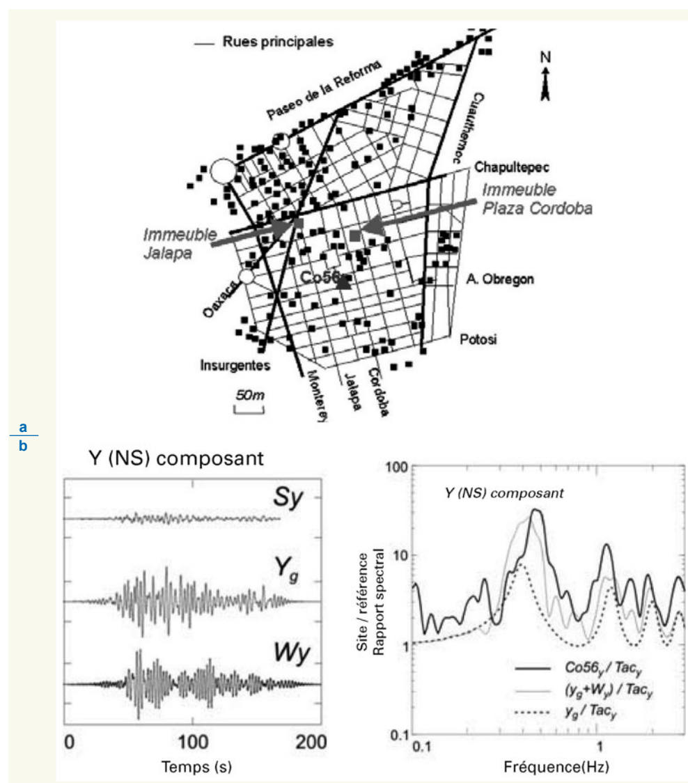
figure 4 Modélisation de l'interaction site-ville du quartier Roma de la ville de Mexico.
