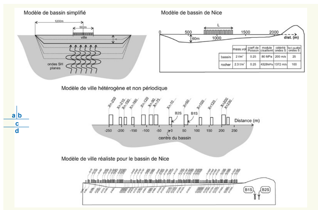
figure 5 Modèles de ville et de bassin pour l'analyse bidimensionnelle de l'interaction site-ville par la méthode des éléments de frontière (Kham et al, 2006 ; Semblat et al, 2008) : a : en haut à gauche : modèle canonique de bassin ; b : en haut à droite : modèle du bassin de Nice ; c : milieu : ville non périodique pour le modèle canonique ; d : en bas : modèle de ville pour Nice. (il faut refaire la figure et la découper pour la numérotter)
