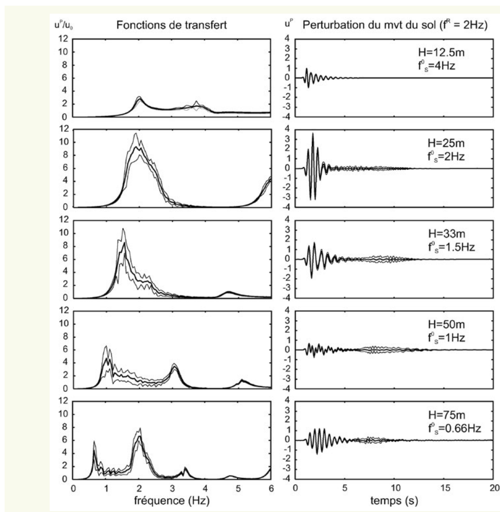
figure 6 Résultats des calculs pour le modèle canonique de ville périodique a : Gauche : fonctions de transfert (moyenne +/- un écart type) pour le modèle canonique de ville périodique (bâtiment B2S) avec N = 33 et différentes valeurs de H (les solutions sont comparées au modèle sans bâtiments en pointillé). b : Droite : perturbation du mouvement du sol dans le cas d'un signal de Ricker de fréquence centrale 2Hz.
