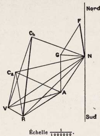
Schéma des triangulations effectuées par Simonin et coll. pour obtenir les distances mont Gros-La Gaude et mont Gros-mont Vinaigre, à partir des positions des piliers géodésiques du premier ordre des monts Cheirojn, mont Féron, du cap Roux et de Nice. (Simonin, in Annales de l'Observatoire de la Côte d'Azur )
