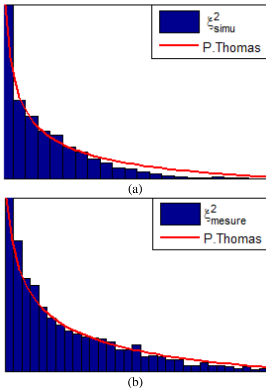
Figure 7. (a) Simulation et (b) mesure de la distribution de |E_z|^2 sur la zone centrale à 3.00GHz. Lois de Porter-Thomas les plus proches.
