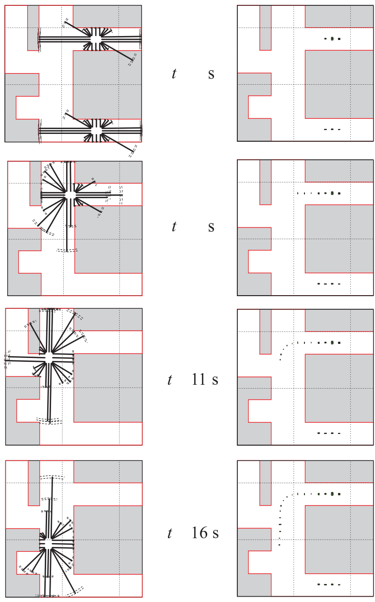
Figure 11: Evolution de deux configurations possibles du robot et projection des ensembles solution sur le plan (x, y) ; à partir de t = 5 s, l'une des deux configurations est jugée incompatible avec les données
