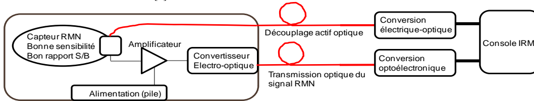
Figure1 : Schéma de la sonde endoluminale à modulation externe électro-optique avec découplage actif
