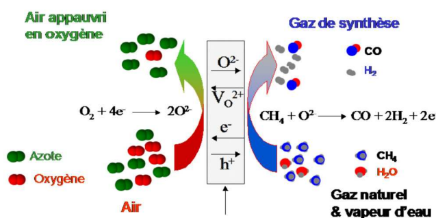
Figure 1. Principe d'une membrane pour la séparation de l'oxygène de l'air, cas d'un réacteur pour reformage du méthane ( V_{\text{O}}^{2+} est une lacune d'oxygène, h^+ est un trou électronique, ce qui correspond à un changement de valence)
