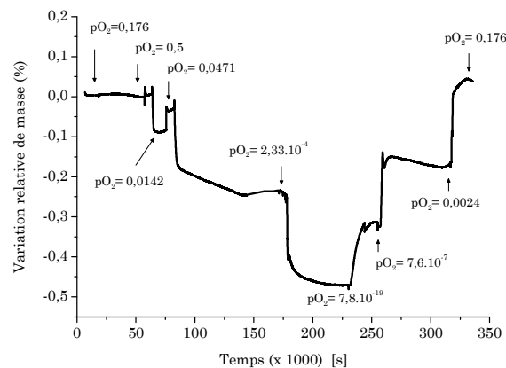
Figure 3. ATG à 900°C sur LSFSG pour différentes atmosphères
