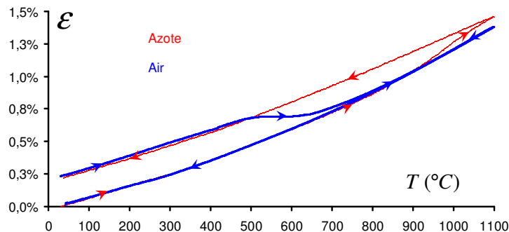
Figure 5. dilatométrie cycle sur LSFG avec changement d'atmosphère
