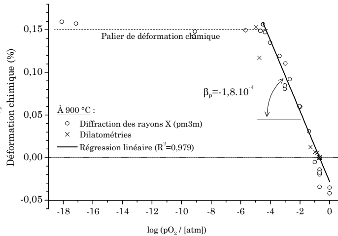
Figure 6. Déformation par DRX de LSF
