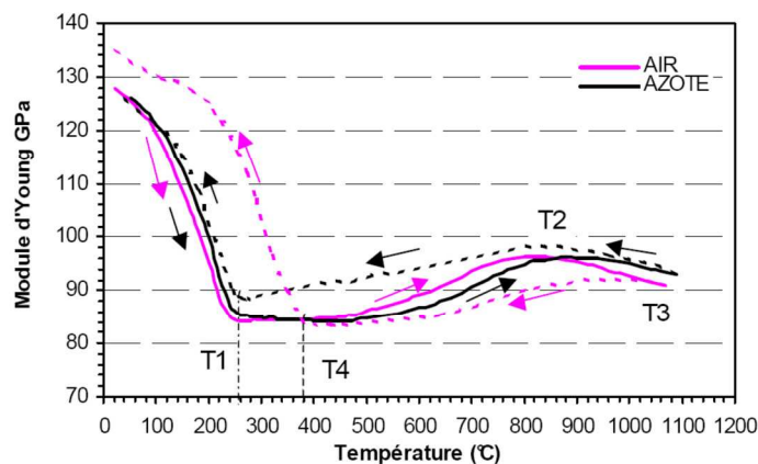
Figure 7. Évolution du module d'Young de LSF en fonction de la température et de l'atmosphère (Julian 09)
