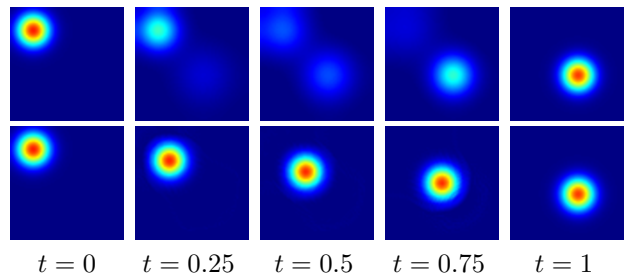
FIGURE 5 – Interpolation entre deux densités. Ligne du haut : chemin géodésique de L^2 . Ligne du bas : chemin géodésique de l'espace de Wasserstein. Distance L^2 = 0.0645 , Distance de Wasserstein = 20.26.
