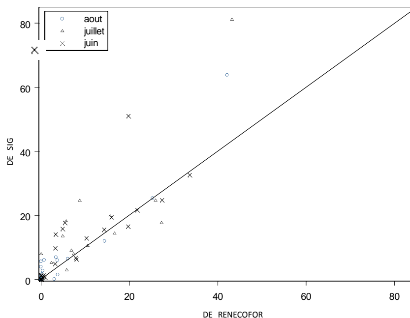
Figure 16 : Comparaison des déficits d'évaporation calculées à partir des données de 25 placettes RENECOFOR pour les mois de juin, juillet et août et extraites du SIG sur ces mêmes placettes ( N = 25 * 3 mois).
