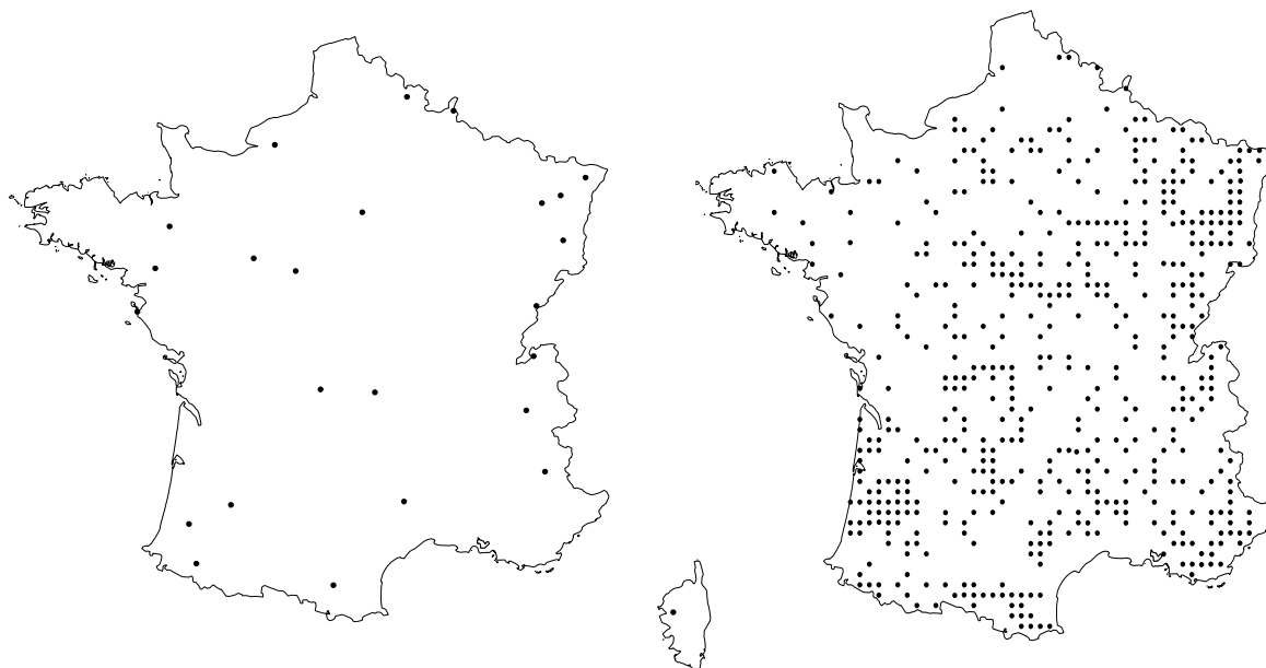
Figure 8 : localisation géographique des 25 placettes du réseau RENECOFOR (à gauche) et des 543 placettes du réseau Biosoil (à droite) utilisées.
