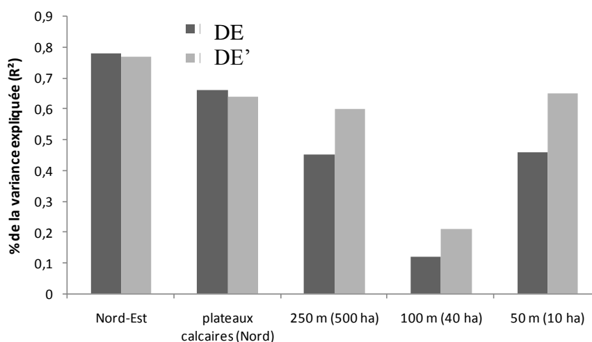
Figure 18 : Part de la variance des déficits d'évaporation estimés sur le terrain expliquée par les cartes numériques de et DE' sur des emprises de taille décroissante (quart nord est de la France, partie centre et nord des plateaux calcaires, maillages de 250 – 100 et 50 m sur la forêt de Bois l'évêque/Villiers le sec).
