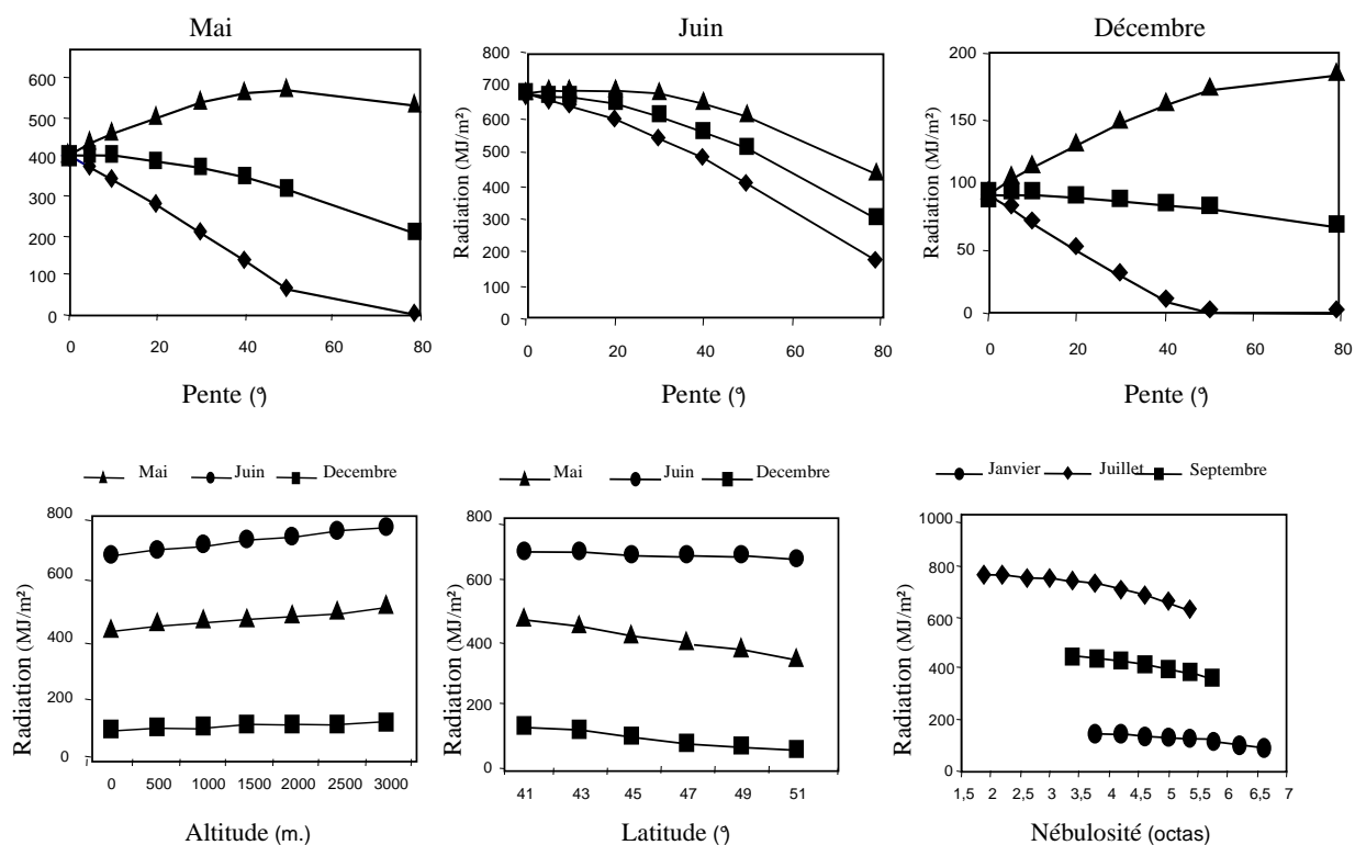
Figure 5. Variations de rayonnement solaire en fonction de l'altitude, de la latitude, et de la nébulosité (MJ/m 2 )
