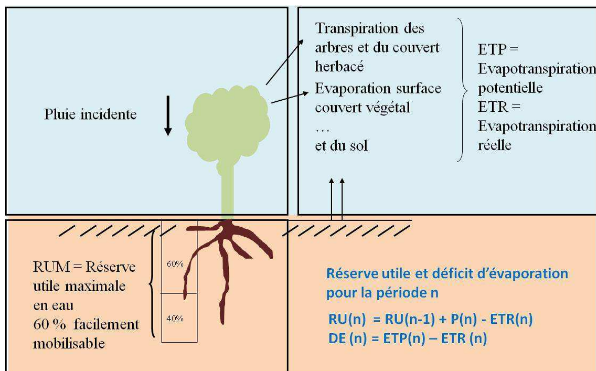
Principe du bilan en eau des sols simplifié utilisé pour calculer les cartes mensuelles de contrainte hydrique.
