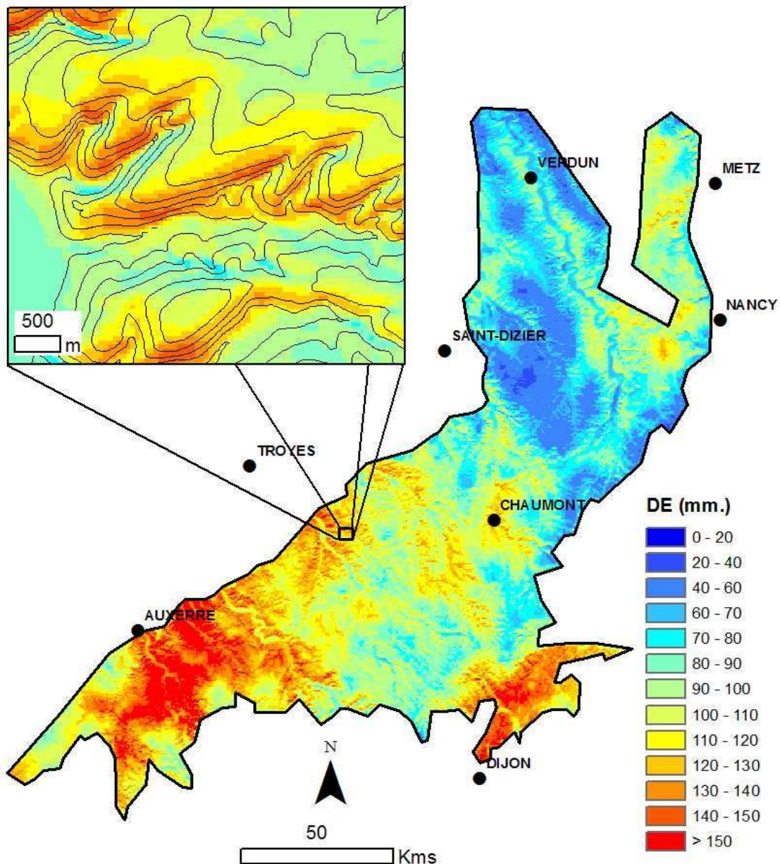
Cartographie du déficit d'évaporation estival (cumul de juin, juillet et août) sur la zone des plateaux calcaires de Lorraine, Bourgogne et Champagne-Ardenne et zoom au 1/50 000ème sur un vallon au sud-est de Troyes. Une valeur de déficit d'évaporation élevée (couleur rouge) indique une plus forte contrainte hydrique.
