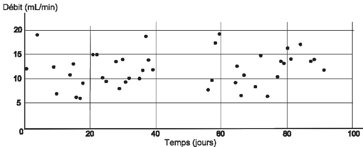
Figure 5. Débit de liqueur à la sortie du mini-drain sous une charge hydraulique de 0,005m.
