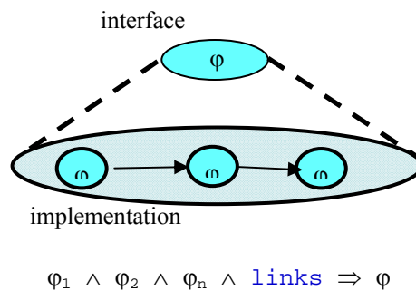
Figure4: BHD Refinement.
