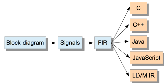
Figure 1. Etapes internes de la compilation dans Faust
