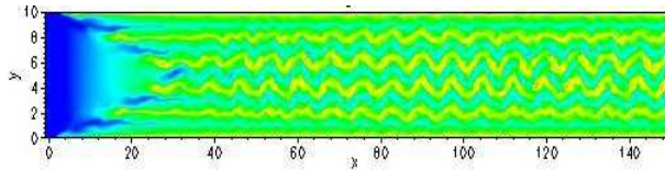
Figure 6 : (au dessus) Champ de température en z=0.5 dans l'écoulement de dix R_z à Re=150 , Ra=14575 ( \epsilon=3,5 ), A_{exc}=2 et f_{exc}=0,16 .
