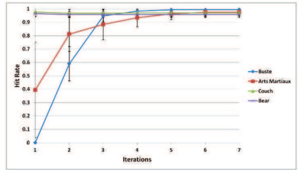
FIGURE 9 – Pour les 4 jeux de données, l'algorithme converge après 6 itérations.
