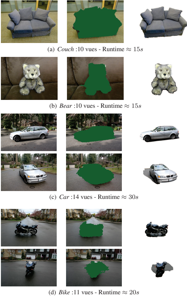
FIGURE 5 – Résultats sur Car et Bike [11]. Les points verts indiquent les échantillons avec p_s^f > 0.8 . La dernière colonne représente le résultat de la segmentation.
