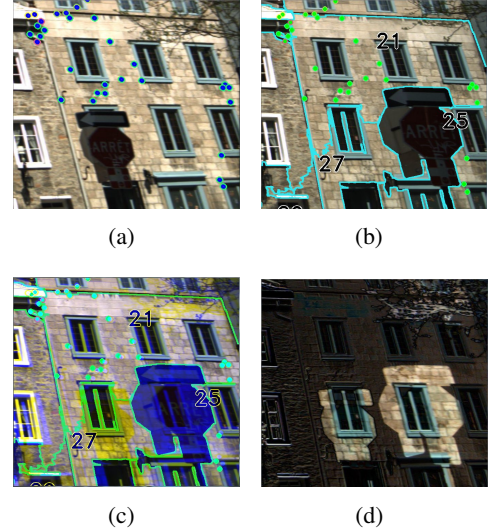
FIGURE 7 – Zoom sur une zone plane. (a) H_0(im_0) zone plane recalée de l'image précédente et (b) im_1 zone plane d'intérêt de l'image centrale. (c) Superposition de ces deux zones ( im_1 est visualisée sur les canaux vert et rouge et H_0(im_0) est représentée sur le canal bleu). (d) Différence sur les trois canaux de couleur entre (a) et (b). Les zones mal recalées sont mises en évidence, comme, par exemple, le panneau.
