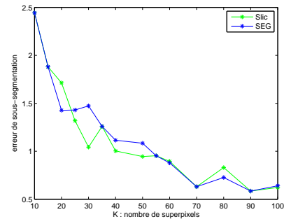
FIGURE 12 – Erreur de sous-segmentation pour c = 10 .
