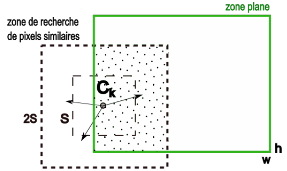
FIGURE 10 – Calcul de la pénalité – Pour chaque pixel de la zone de recherche centrée sur C_k qui appartient à une zone plane, la pénalité d_{plan} est prise en compte.
