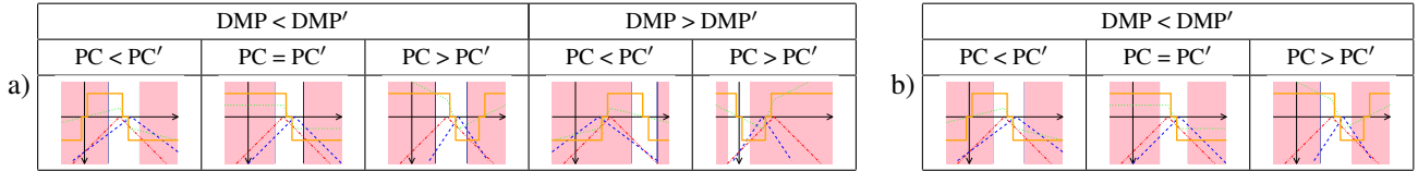
FIG. 5 – a) Candidats possibles pour l'exemple où C(d) change de positive à négative dans la partie visible de la disparité (intervalle non-rayé) : 5 configurations possibles. b) Candidats possibles si on suppose que les disparités correspondantes aux DMP des deux caméras sont dans l'intervalle de disparité mesurable (intervalle non-rayé) : plus que 3 configurations possibles.
