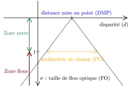
FIG. 1 – Le modèle de flou dû à l'optique : la taille du FO est une fonction de la disparité stéréoscopique linéaire par morceaux. Elle est nulle à la disparité correspondante à la distance de mise au point (DMP) et sa pente est inverse à la profondeur de champ (PC).
