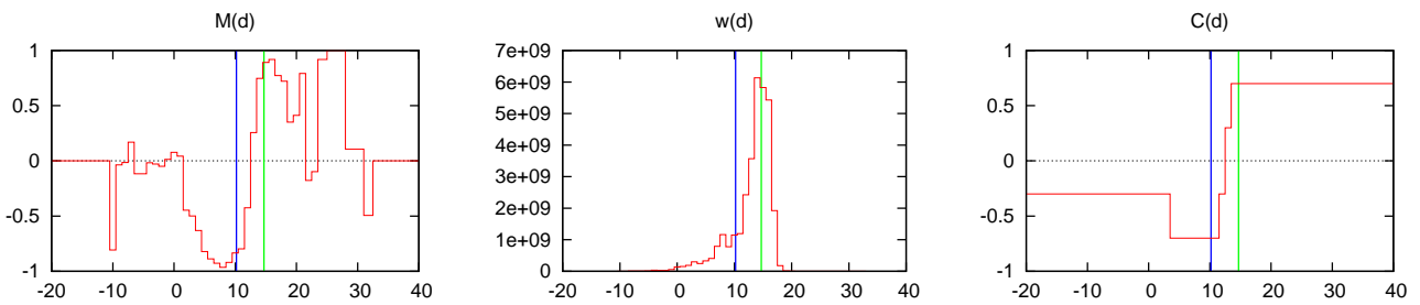
FIG. 8 – Résultats pour la paire ( GLoin, DPrès ). De gauche à droite : M(d) : moyenne pondérée du signe de la différence de SML. w(d) : somme du maximum des valeurs de SML. C(d) : Modèle estimé. Les disparités bleu et verte correspondent aux disparités Près et Loin .
