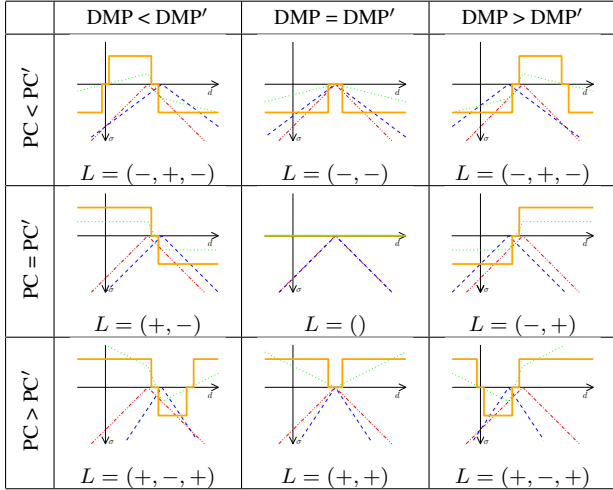
FIG. 3 – Catalogue des types de courbes possibles pour chaque configuration. En orange, le signe de la différence de FO. En pointillées les fonctions de FO gauche (rouge), FO droite (bleu) et leur différence (vert). Pour chaque courbe nous donnons aussi la liste L de signes que nous utiliserons dans la méthode de classification (Sec 3.5).
