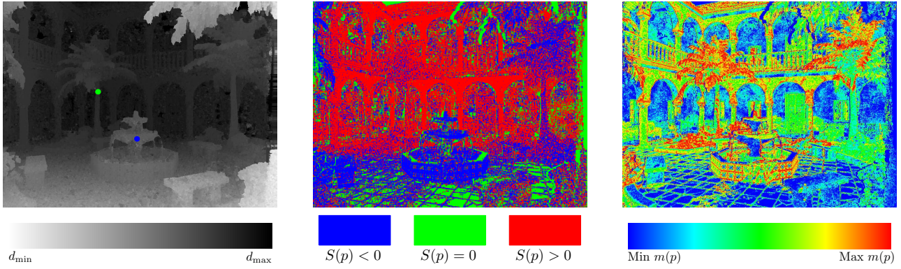
FIG. 7 – Résultats intermédiaires pour la paire ( GLoin, DPrès ). De gauche à droite : d(p) : Disparité calculée. S(p) : Signe de la différence de SML. m(p) : Maximum des SML. Les points bleu et vert dans la carte de disparité correspondent aux DMP Près et Loin .
